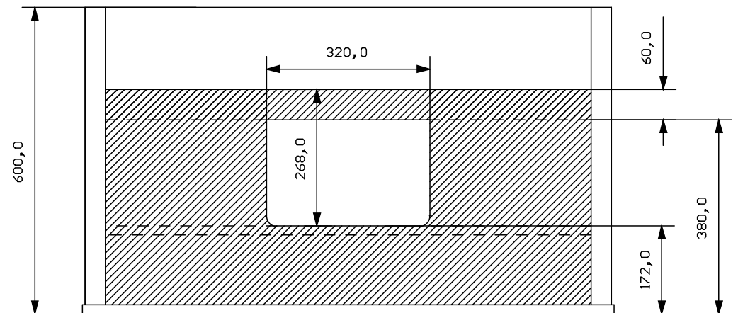
vista posteriore
