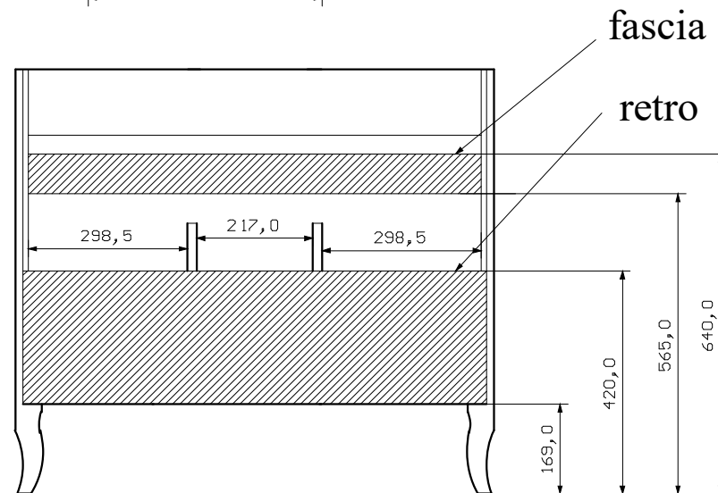
vista posteriore
