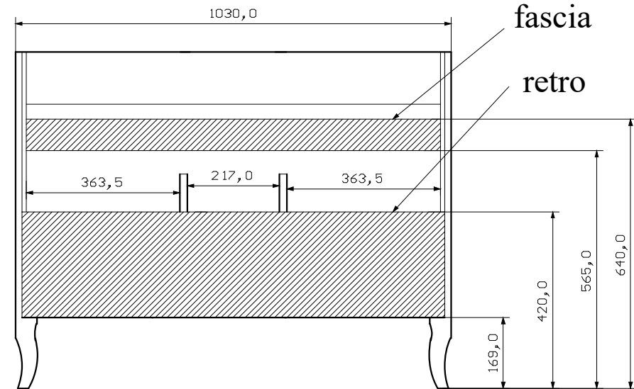
vista posteriore
