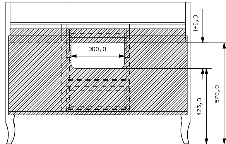
vista posteriore
