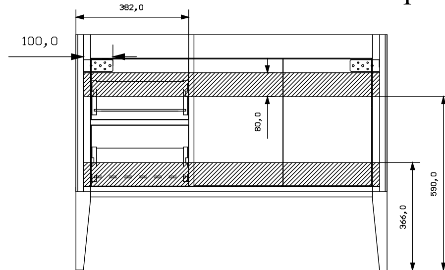
vista posteriore
