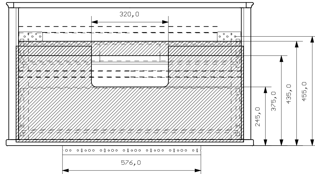
vista posteriore
